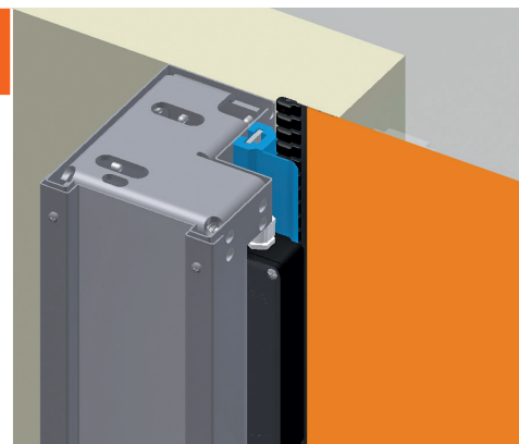
Selbsttestender SLE-Mechanismus
