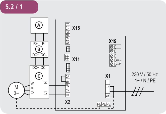
Detailschaltplan Netzanschluss und Motoranschluss (230V / 1-phasig / 0,75 kW)
