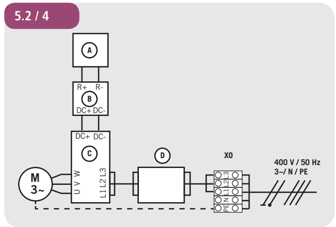
Detailschaltplan Netzanschluss und Motoranschluss (400 V / 3-phasig / 4,0 kW)
