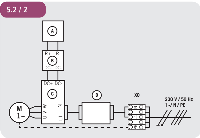
Detailschaltplan Netzanschluss und Motoranschluss (230V / 1-phasig / 1,5 kW)
