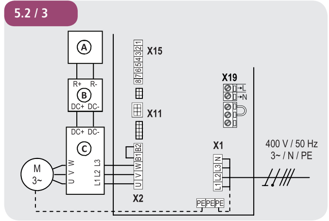
Detailschaltplan Netzanschluss und Motoranschluss (400 V / 3-phasig / 1,5 kW / 2,2 kW / 3,0 kW)
