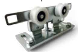
Laufwagen mit Rollen aus Technopolymer Dupont™ Delrin® und Entgleisungsschutzsystem
